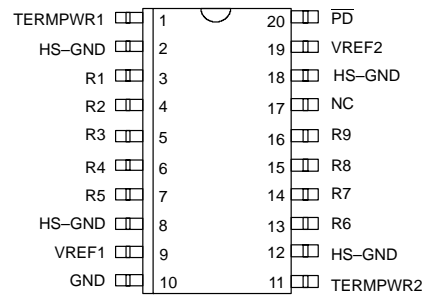
DS2107AE 20-Pin TSSOP (173 mil)
